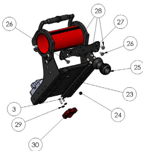
Exploded view van de centrale unit met electronica
