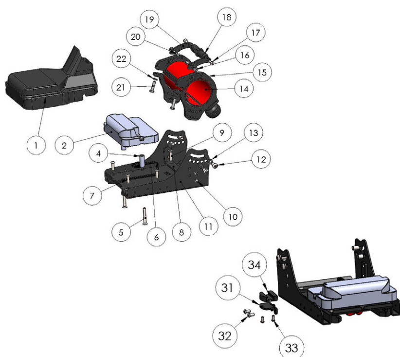
Exploded view van de centrale unit met electronica
